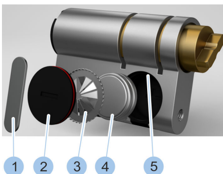
Abb. 148: Batterien wechseln
