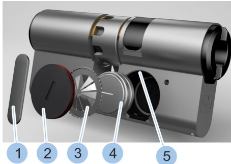
Abb. 127: Batterien entnehmen
