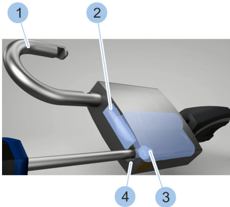
Abb. 146: Befestigungsschraube lösen
