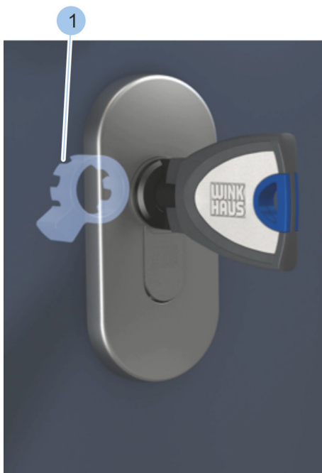
Abb. 36: Schließbart ausrichten
