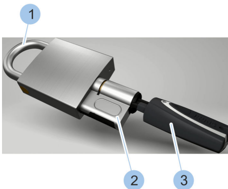
Abb. 147: Zylinder herausziehen
