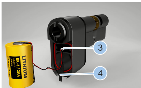
Abb. 141: Batterie entnehmen
