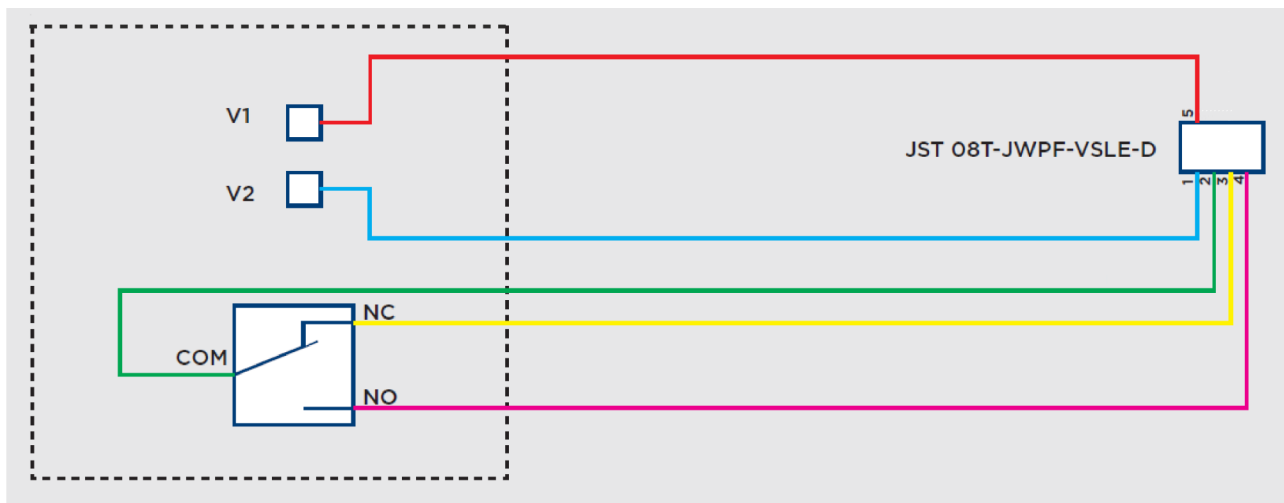
Abb. 48: Relaisverkabelung
