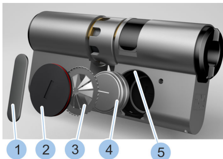
Abb. 128: Batterien einlegen
