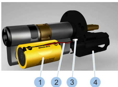
Abb. 136: Batterie einsetzen
